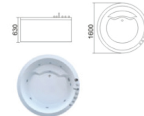
TF-BT-232 ממ 1600 x 1600 x 630
