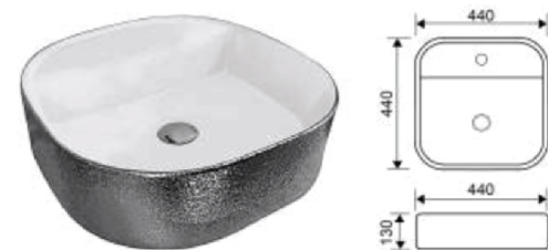
TF-OTWB-110-S อ่างล้างหน้าวางบนเคาน์เตอร์ ขนาด 440 x 440 x 130 มม. เคลือบสีเงิน
