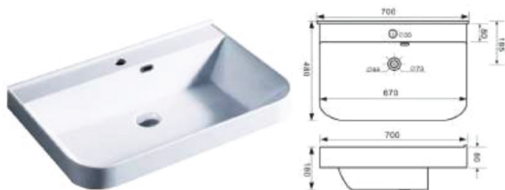
TF-UCWB-503 อ่างล้างหน้าฝังบนเคาน์เตอร์ ขนาด 600 x 400 x 150 มม. วัสดุ หินสังเคราะห์
