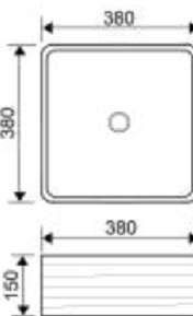
TF-OTWB-165-GR อ่างล้างหน้าวางบนเคาน์เตอร์ ขนาด 380 x 380 x 150 มม. สีเทา
