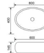
TF-OTWB-180 อ่างล้างหน้าวางบนเคาน์เตอร์ ขนาด 600 x 400 x 145 มม. เคลือบสีทอง
