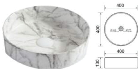
TF-OTWB-235 อ่างล้างหน้าวางบนเคาน์เตอร์ ขนาด 400 x 400 x 130 มม. แบบไม่มีรูน้ำล้น
