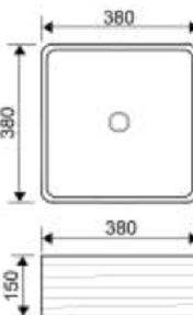
TF-OTWB-165-B อ่างล้างหน้าวางบนเคาน์เตอร์ ขนาด 380 x 380 x 150 มม. สีดำ
