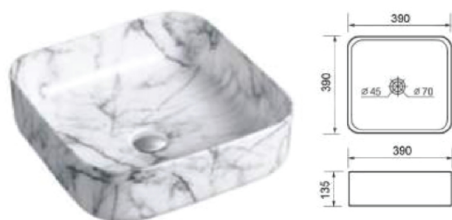
TF-OTWB-236 อ่างล้างหน้าวางบนเคาน์เตอร์ ขนาด 390 x 390 x 135 มม. แบบไม่มีรูน้ำล้น
