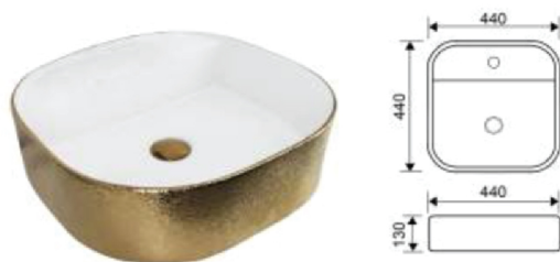
TF-OTWB-110-G อ่างล้างหน้าวางบนเคาน์เตอร์ ขนาด 440 x 440 x 130 มม. เคลือบสีทอง
