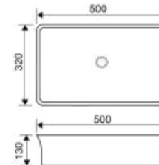
TF-OTWB-125-B อ่างล้างหน้าวางบนเคาน์เตอร์ ขนาด 500 x 320 x 130 มม. สีดำ
