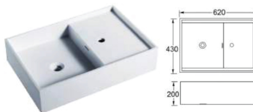
TF-OTWB-520 อ่างล้างหน้าวางบนเคาน์เตอร์ ขนาด 620 x 430 x 200 มม. วัสดุ หินสังเคราะห์
