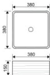
TF-OTWB-165-W อ่างล้างหน้าวางบนเคาน์เตอร์ ขนาด 380 x 380 x 150 มม. สีขาว
