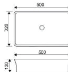
TF-OTWB-125-W อ่างล้างหน้าวางบนเคาน์เตอร์ ขนาด 500 x 320 x 130 มม. สีขาว
